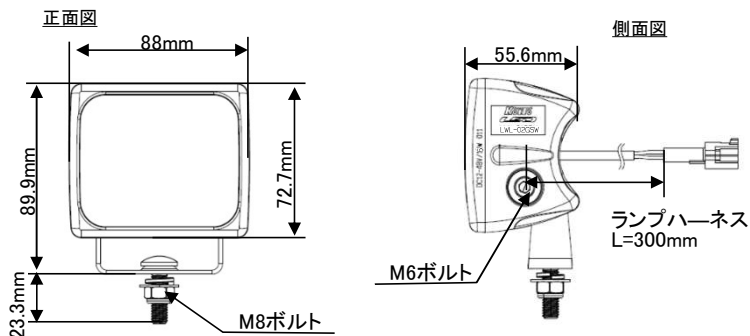
【寸法図】
