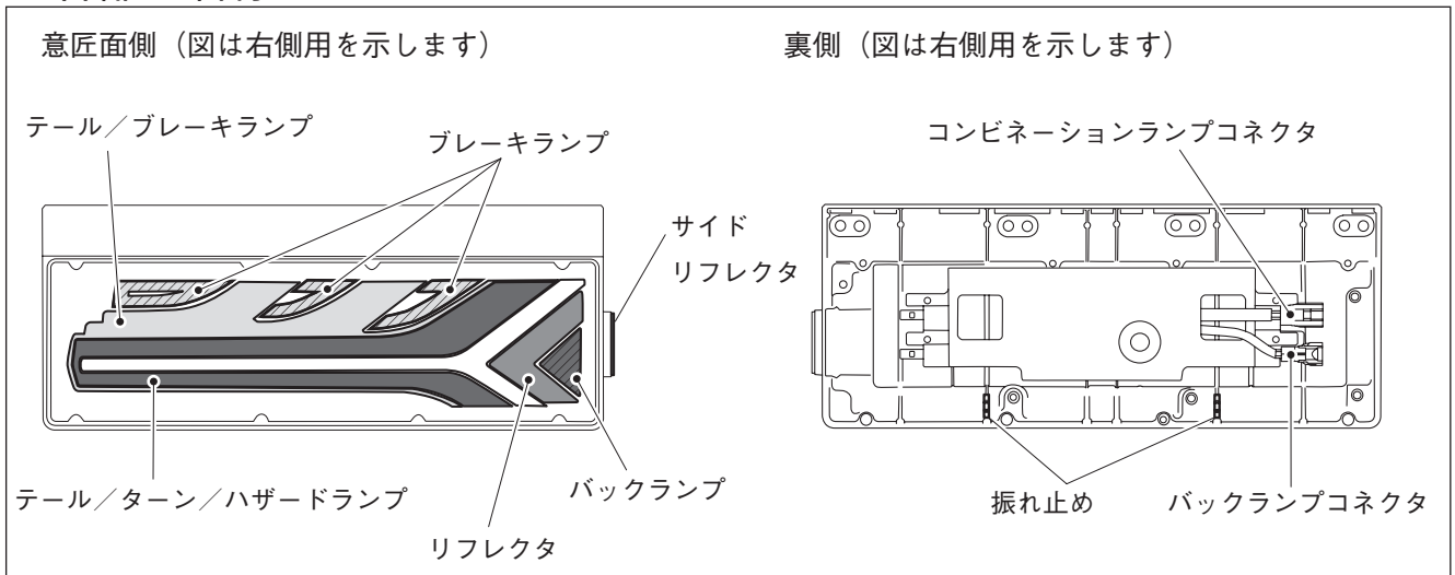
LEDリアコンビネーションランプ 寸法図（単位：mm）
