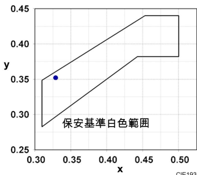
保安基準で求められる白色光の色度範囲
